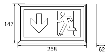
Maße LM Wand
