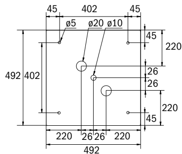
Bohrabstände WX
