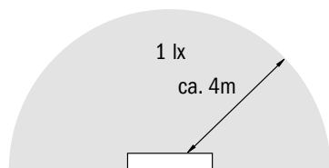
WEF Lichtverteilung
