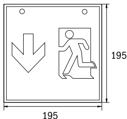
Maße WK
