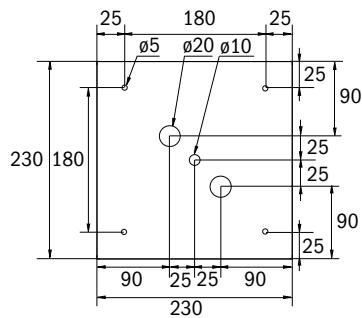
Bohrabstände WX
