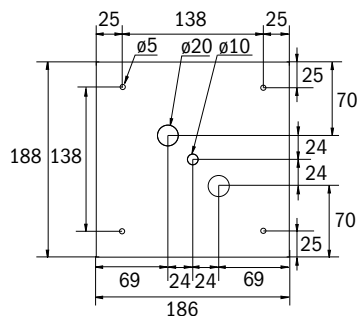
Bohrabstände WK
